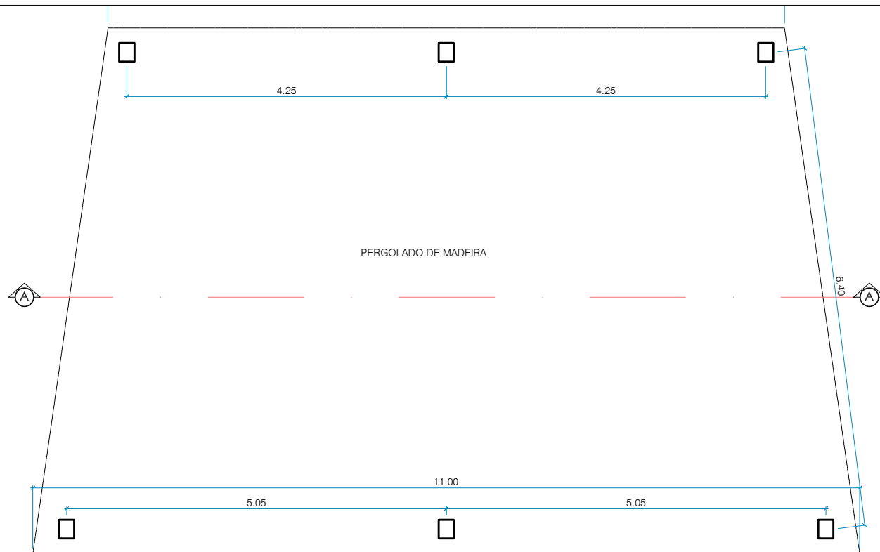
DETALHE 04 COBERTA PLAYGROUND ESCALA: 1/50
